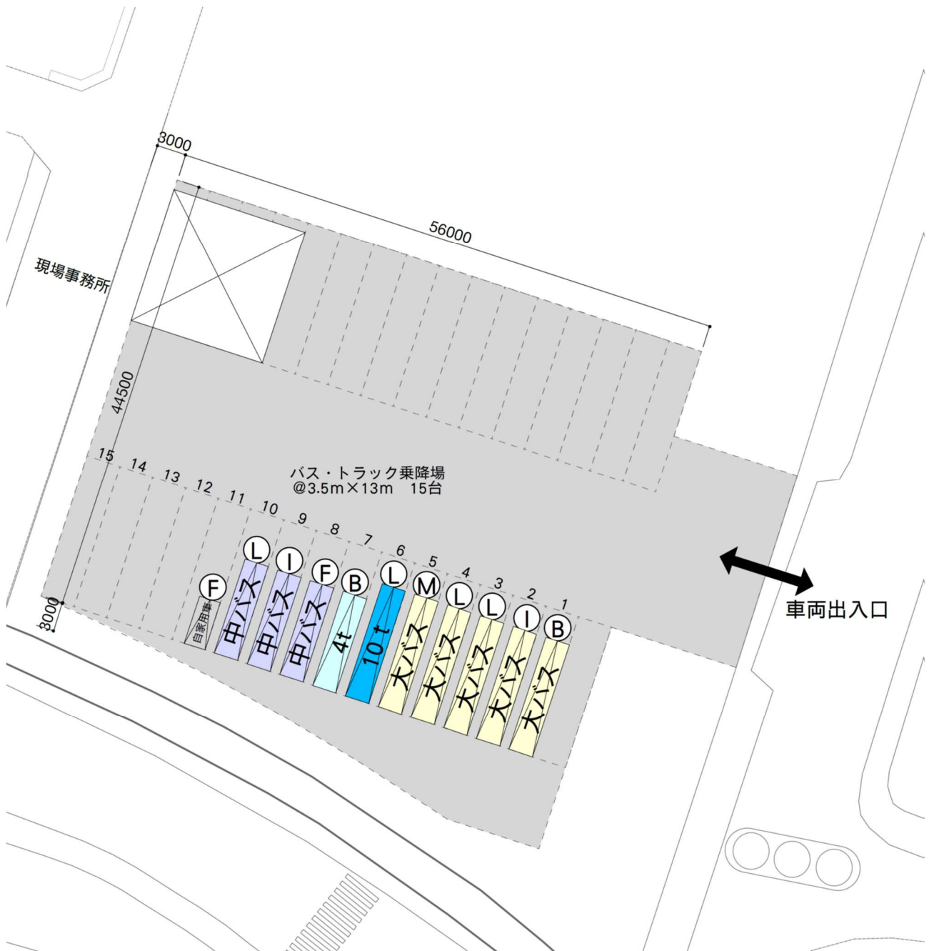
搬出場所（城内中学校跡地）の駐車計画図
